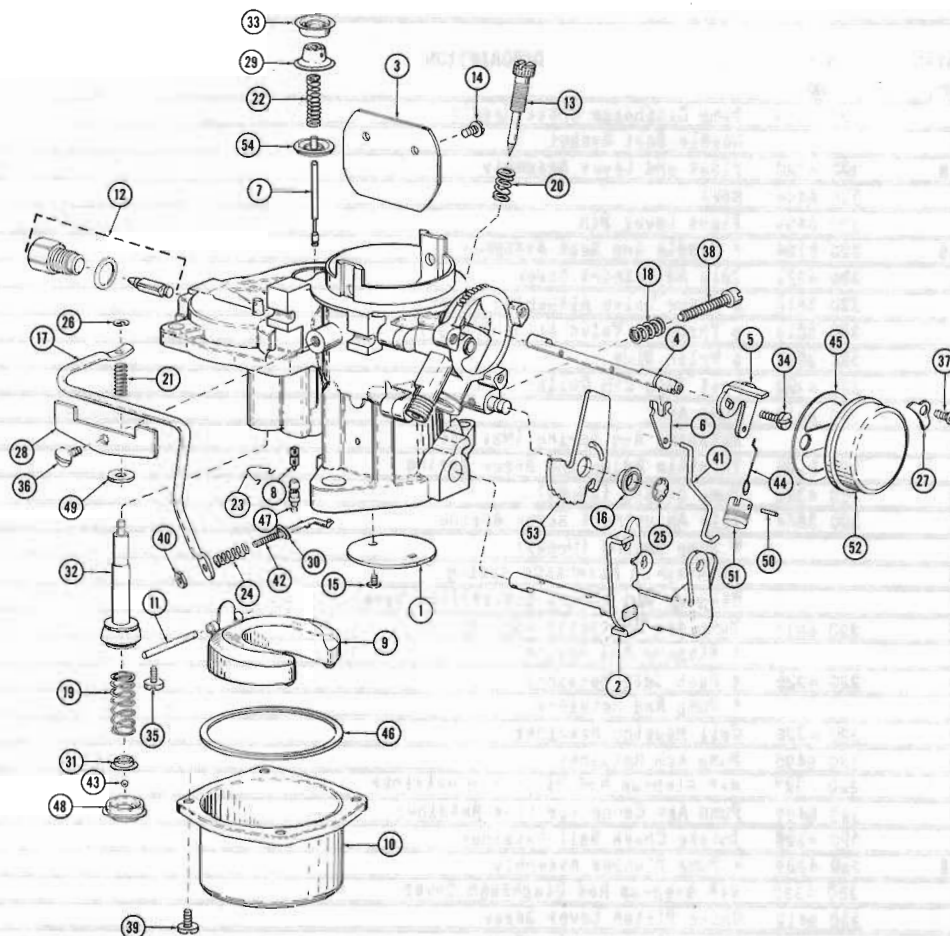
CARBURETOR 64 10 (OHV-196-WAT-LDT)
