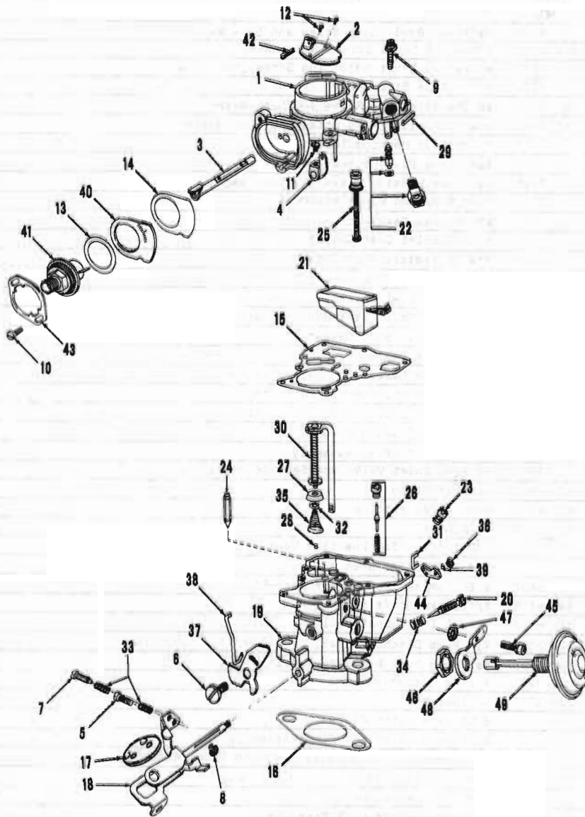
CARBURETOR 63-64 01 (OHV-LDT)
