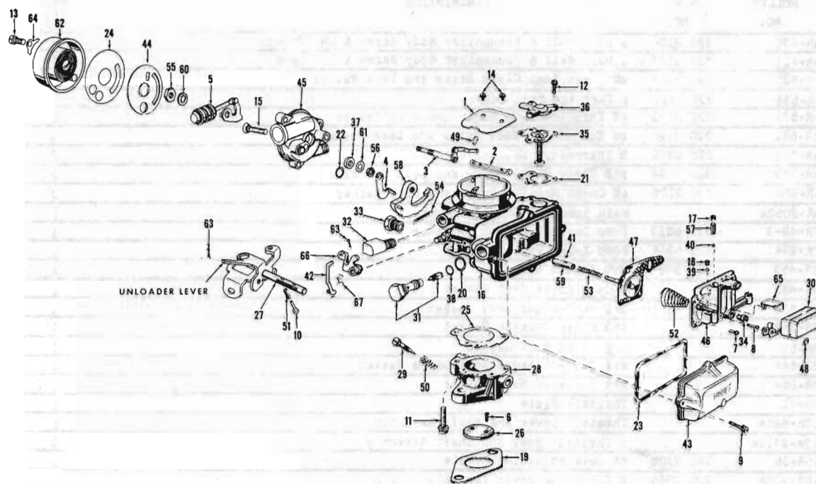
CARBURETOR 61 01 (OHV)
